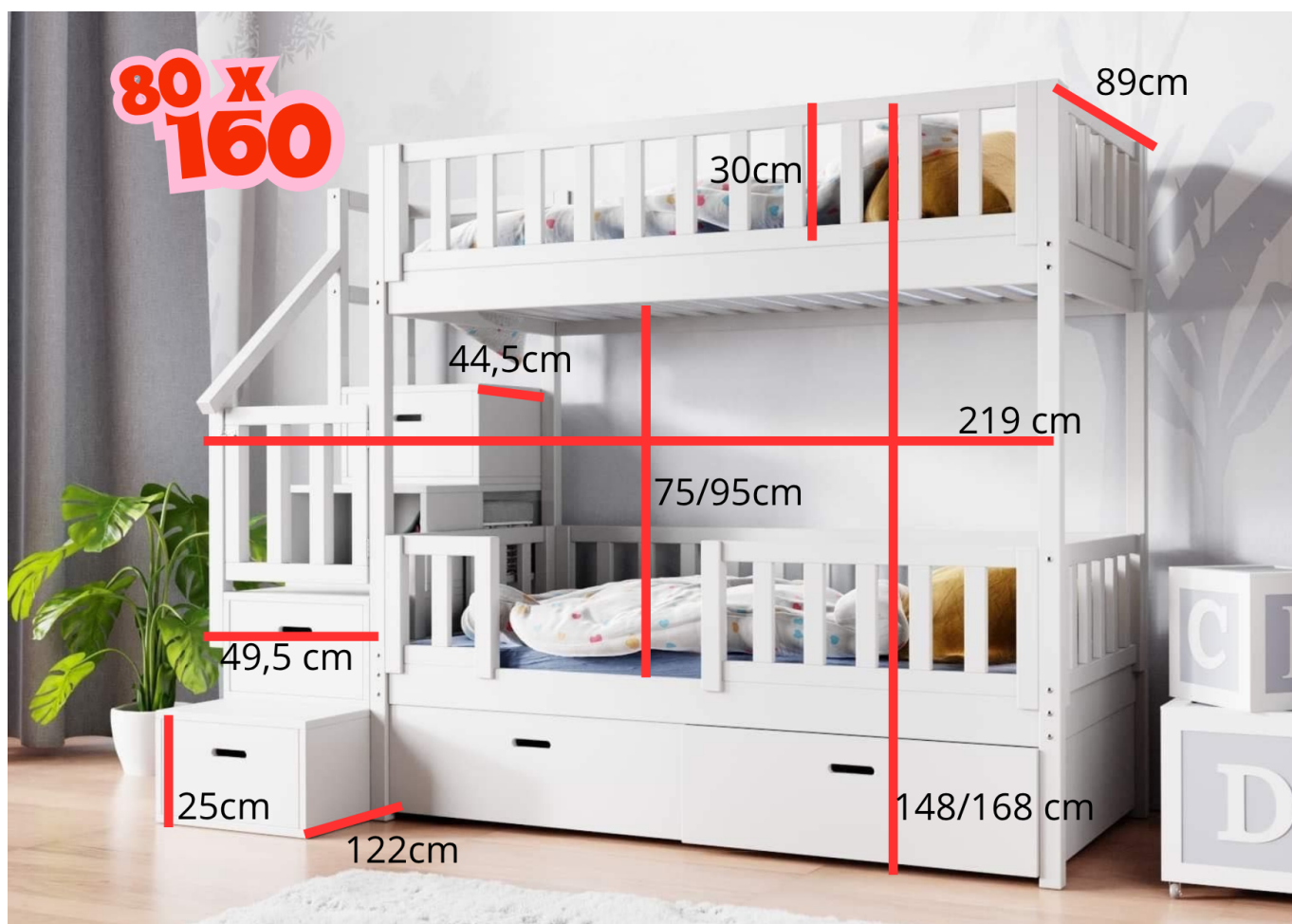
Etagenbett 80x1600
