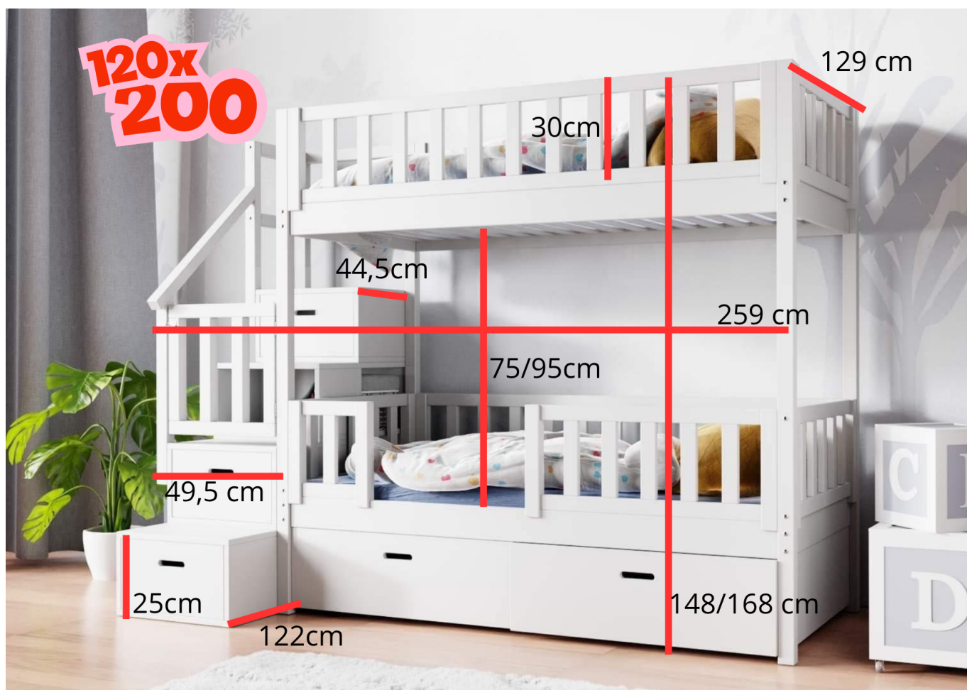
Abmessungen des Etagenbetts mit Treppe
